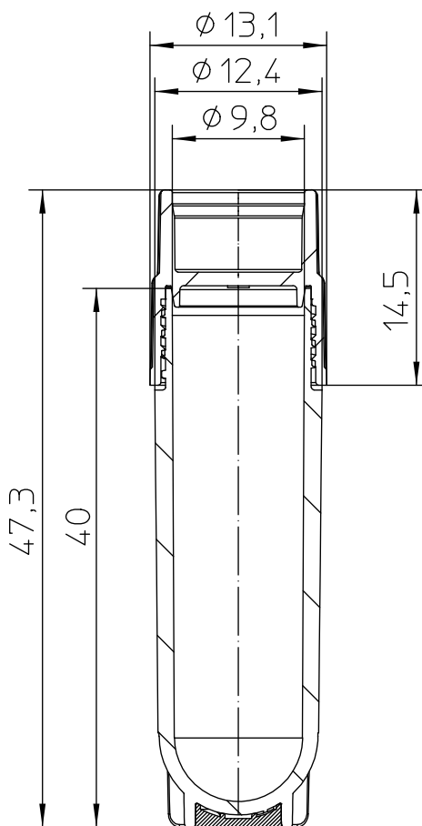
Schnitt A-A
